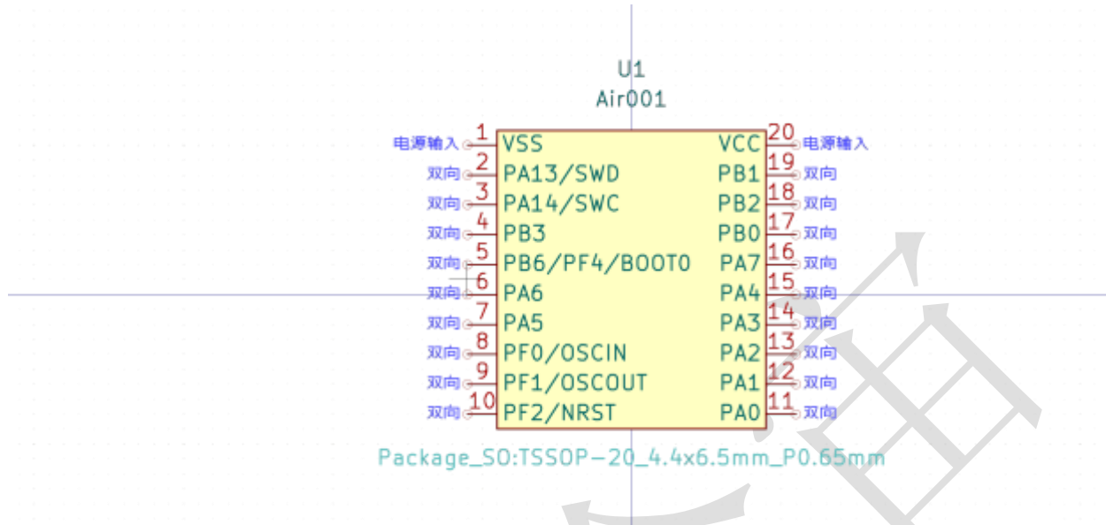
图 1 TSSOP20封装
